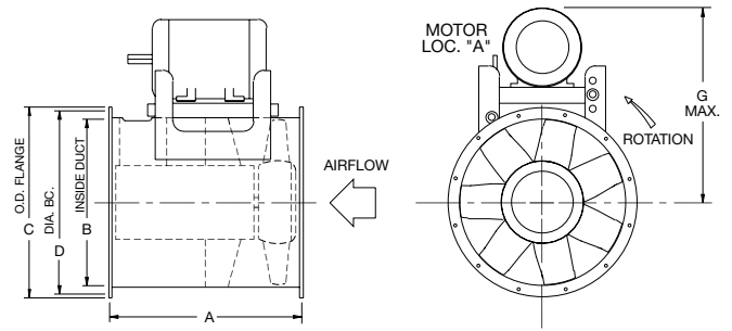
ARR. 9 – HORIZONTAL
