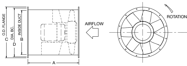
ARR. 4 – HORIZONTAL
