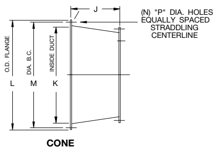
CONE
