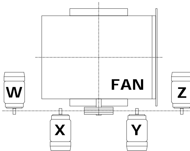
Fig. 3 – Motor Position
