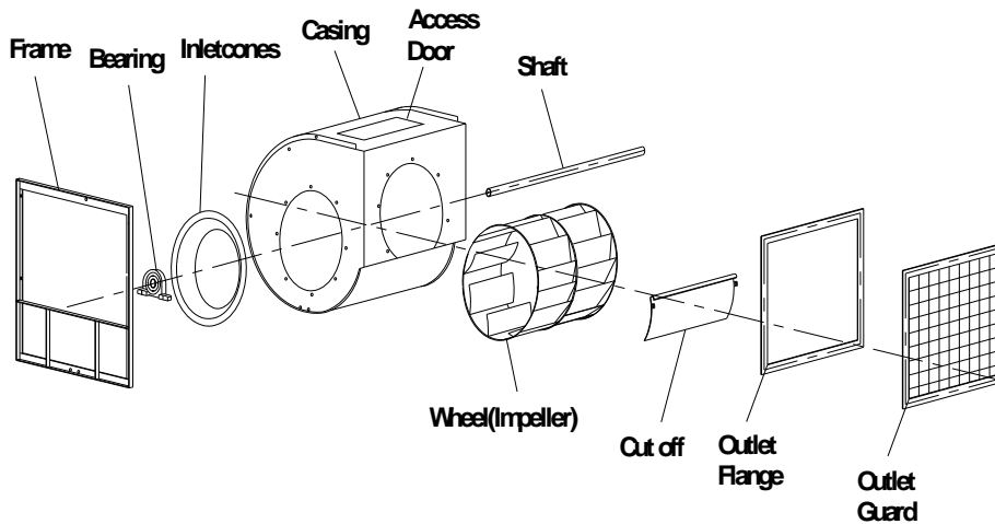
Fan layout drawing
