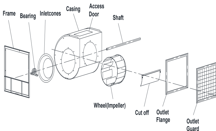
Fan layout drawing
