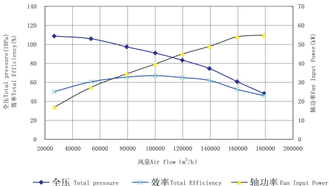
4-79-20E性能曲线图 (Performance curve) n=420r/min
