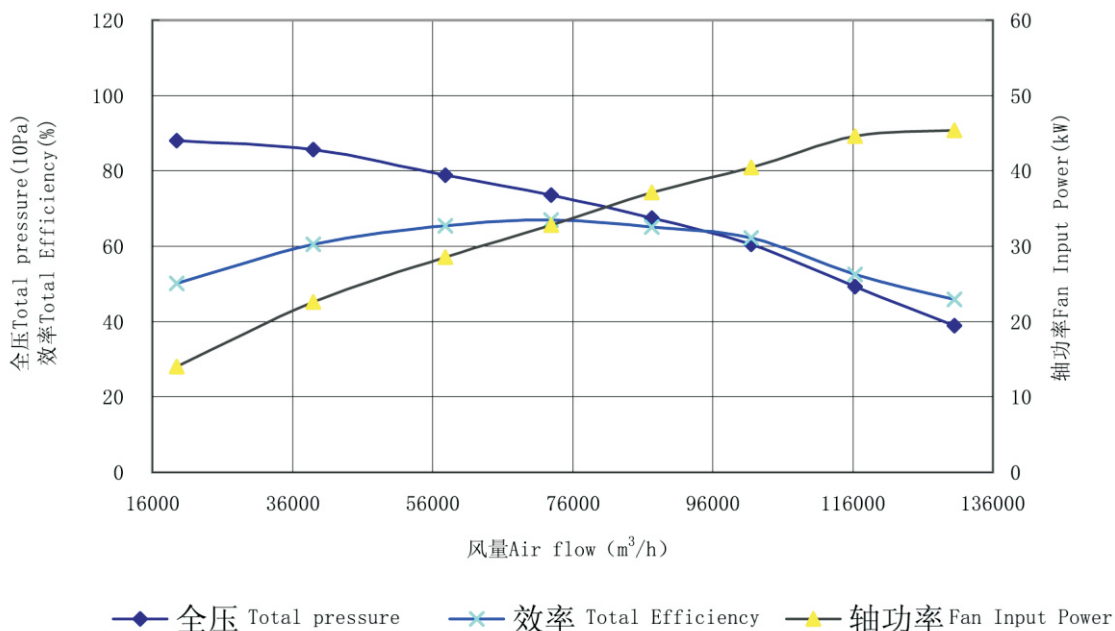
4-79-18E性能曲线图 (Performance curve) n=420r/min
