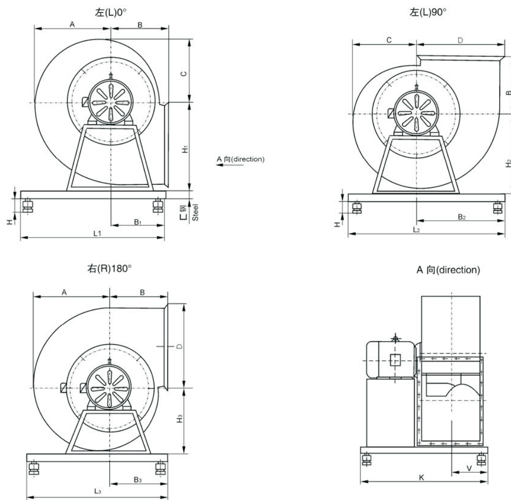
4-79 №3、3.5、4、4.5、5、6 带整体支架外形尺寸 Contour Dimensions with Entirety Rack
