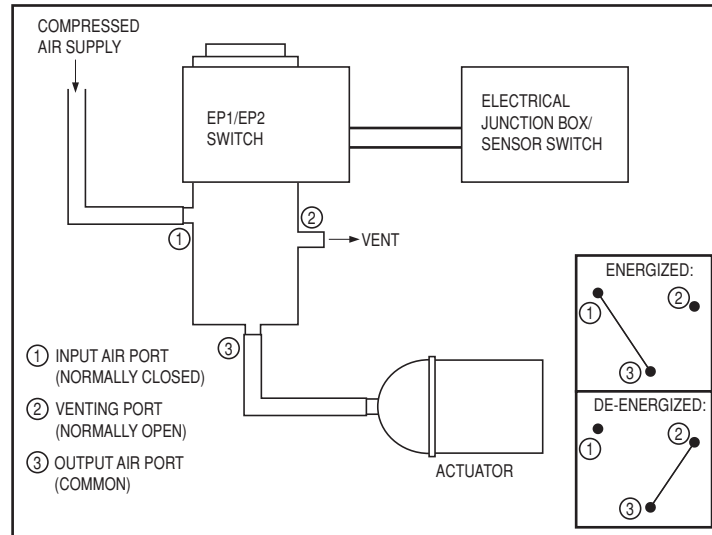
EP1 Siemens 265-1008 120 V/60 Hz EP2 Siemens 265-1007 24 VAC
