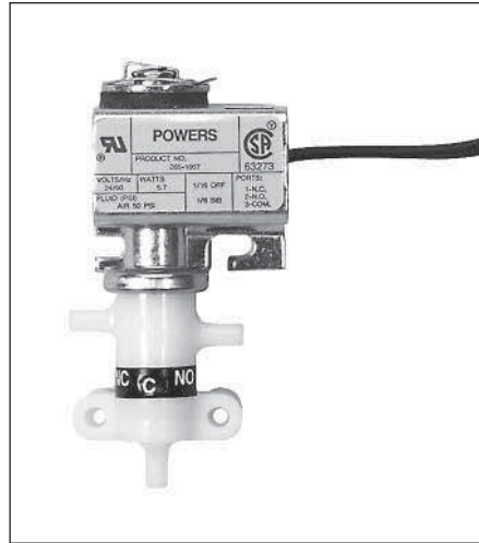
EP1 Siemens 265-1008 120 V/60 Hz EP2 Siemens 265-1007 24 VAC
